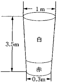
図2 吹流し
